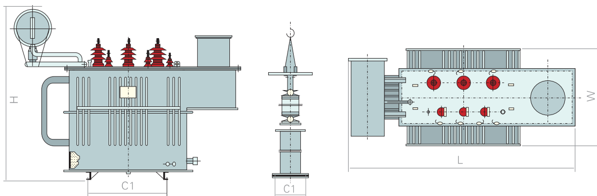
SZ9-200~1600/10变压器
